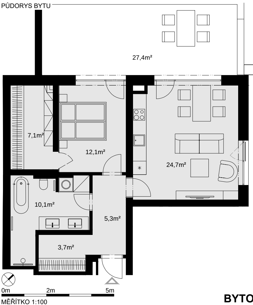
PŮDORYS BYTU
